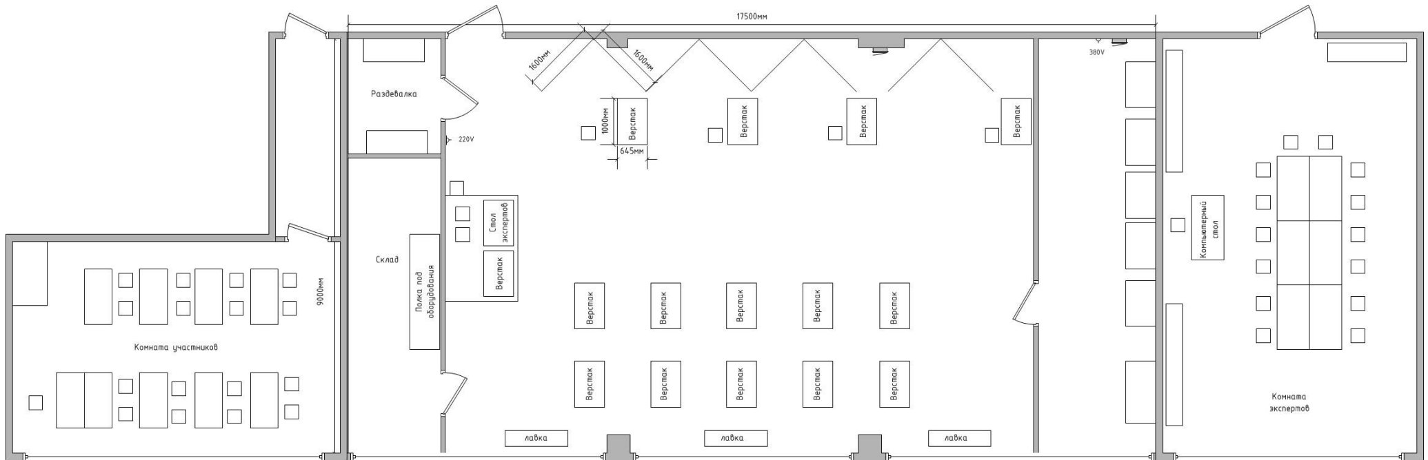
План застройки площадки компетенция электромонтаж – юниоры
